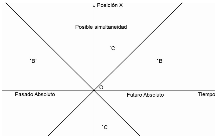
Figura 2. REPRESENTACIÓN DEL ESPACIO-TIEMPO DE MINKOWSKY
